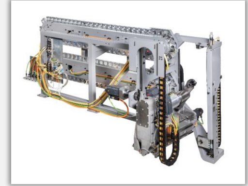
Einbaufertige Systeme
