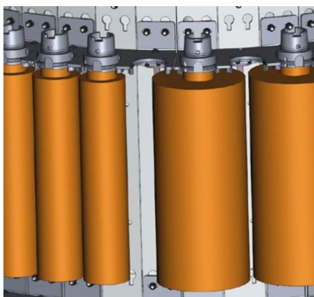
Aufteilung für HSK63, PSC 63, SK40, BT40: Links: Standarddurchmesser bis 80 mm Rechts: Durchmesser bis 160 mm bei freien Nebenplätzen Gewichte: bis 15 kg
