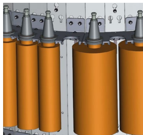
Aufteilung für HSK100, PSC 100, SK50, BT50: Links: Standarddurchmesser bis 125 mm Rechts: Durchmesser bis 280 mm bei freien Nebenplätzen Gewichte: bis 35 kg
